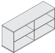
DOUBLE UTILITY TOP FILER UNIT GS1602 + [FINISH] 1600 (W) x 450 (D) x 706 (H)
